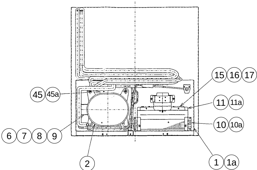
VIEW A-A
